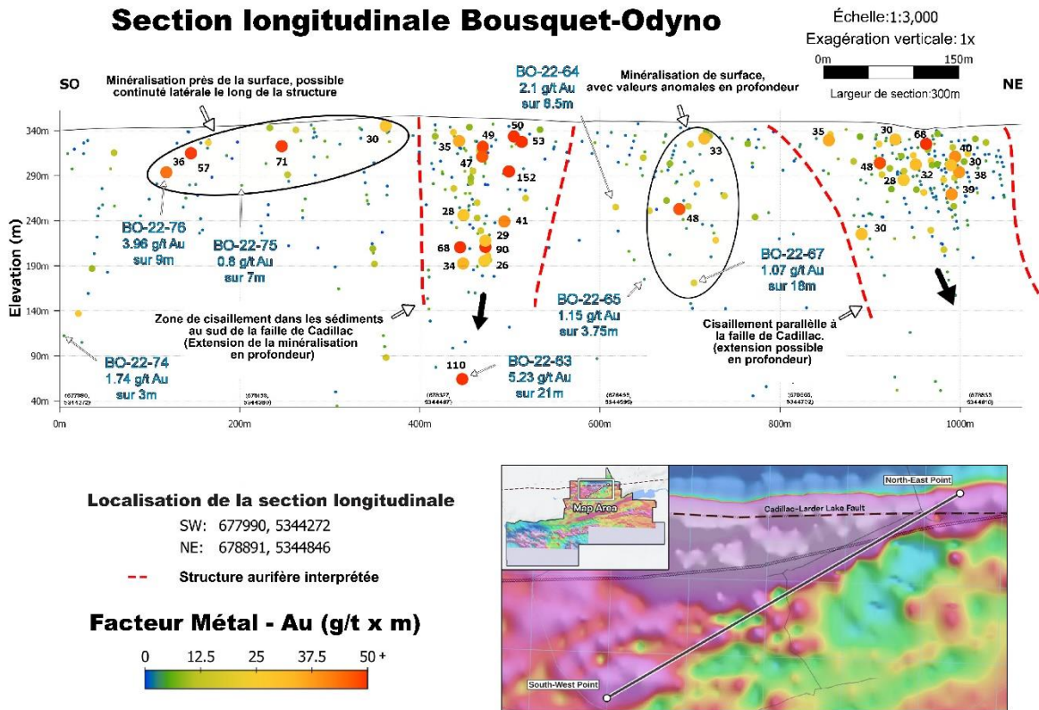
Figure 1 : Section longitudinale du projet Bousquet-Odyno indiquant l'emplacement des sondages.
